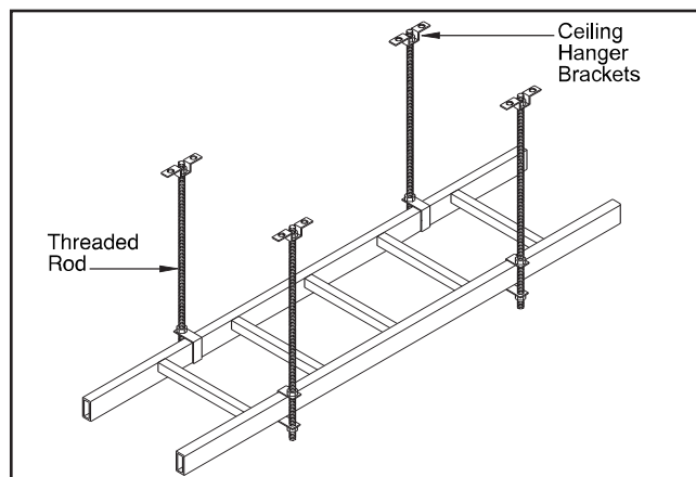
Figure 2—Suspended cable tray (tubular)
