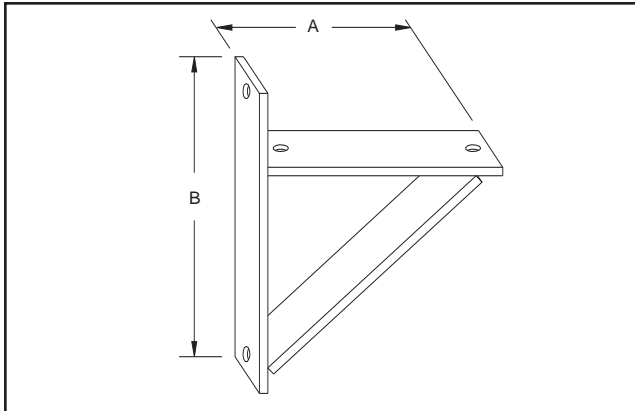
Figure 3—Wall bracket support (tubular)
